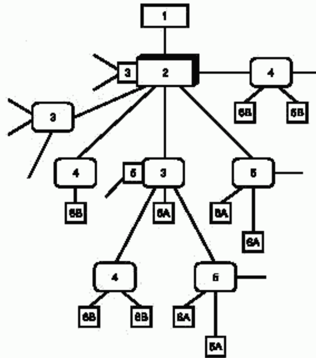
Рисунок F.1 — Большие строительные площадки
