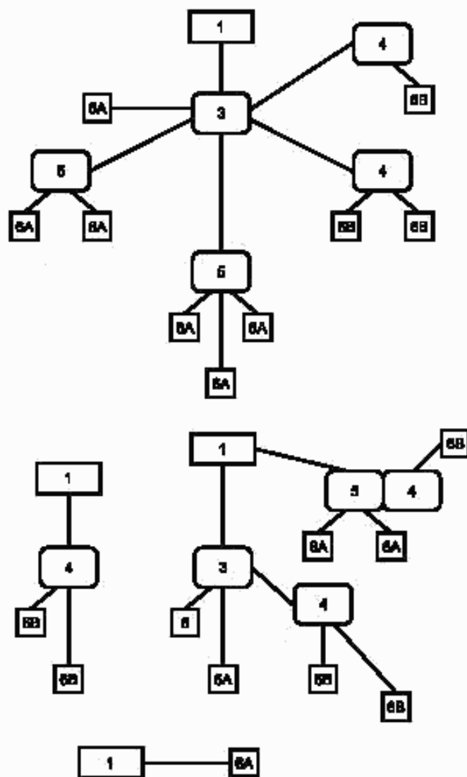
Рисунок F.2 — Средние и небольшие строительные площадки
