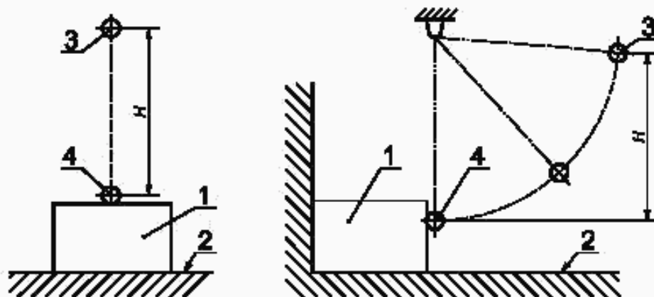
1 — испытуемый образец; 2 — твердая опорная поверхность; 3 — шар в исходном положении; 4 — шар в момент удара
