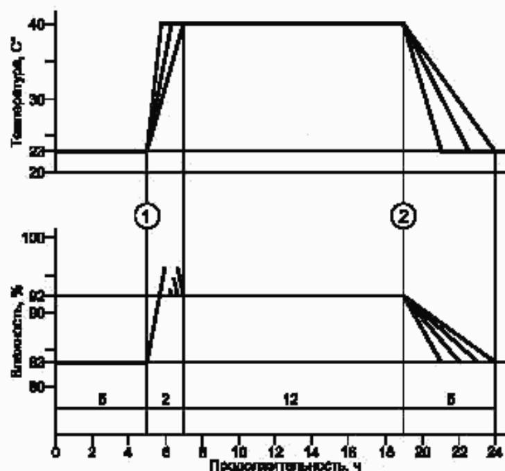
Рисунок 2 — Изменения температуры и влажности по циклам
